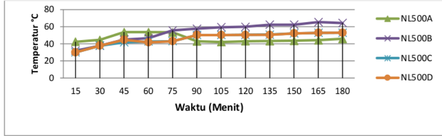
Gambar 13. Grafik hasil pengukuran temperatur (°C) pada sirip lampu.
