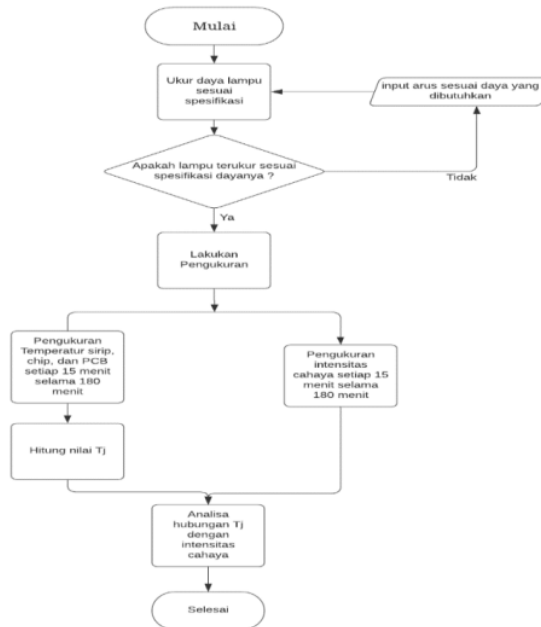
Gambar 4. Diagram alir proses pengukuran lampu.
