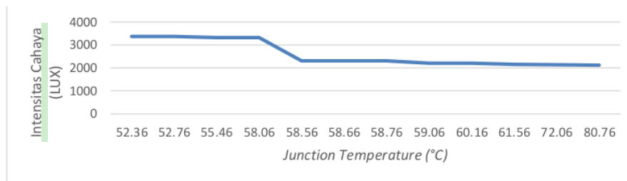
Gambar 6. Grafik pengukuran intensitas cahaya terhadap suhu NL500A.
