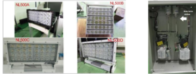
Gambar 3. Model skematik lampu NL500A, NL500B, NL500C, dan NL500D (kiri) dan Metal Halide (kanan).
