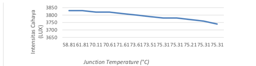
Gambar 12. Grafik pengukuran intensitas cahaya terhadap suhu NL500D.
