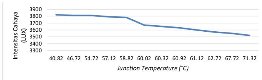
Gambar 10. Grafik pengukuran intensitas cahaya terhadap suhu NL500C.
