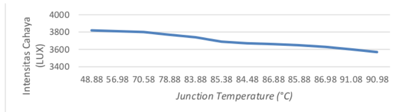
Gambar 8. Grafik pengukuran intensitas cahaya terhadap suhu sambungan NL500B
