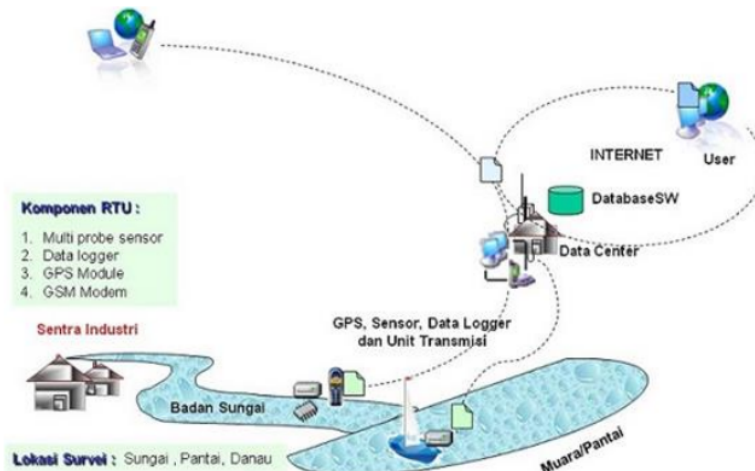
Gambar 2. Skematik sistem pemantauan kualitas air onlino Sumber: [22]
