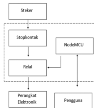
Gambar 1. Diagram Blok Rancangan Perangkat Keras
